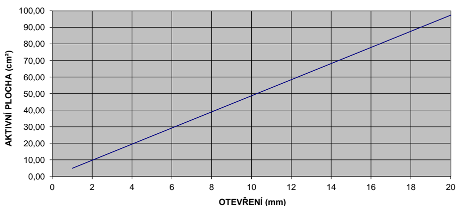
GRAF ZÁVISLOSTI HODNOTY AKTIVNÍ VENTILAČNÍ PLOCHY NA HODNOTĚ OTEVŘENÍ PRO TV Ø 125
