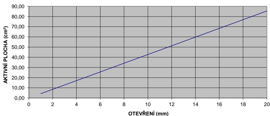
GRAF ZÁVISLOSTI HODNOTY AKTIVNÍ VENTILAČNÍ PLOCHY NA HODNOTĚ OTEVŘENÍ PRO TV Ø 125
