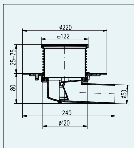
VH – Vodní protizápachová hladina (do interiéru)
